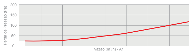
Curva de Perda de Pressão
