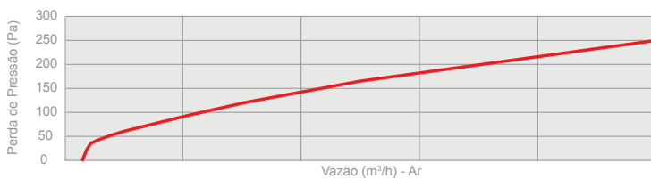
Curva de Perda de Pressão
